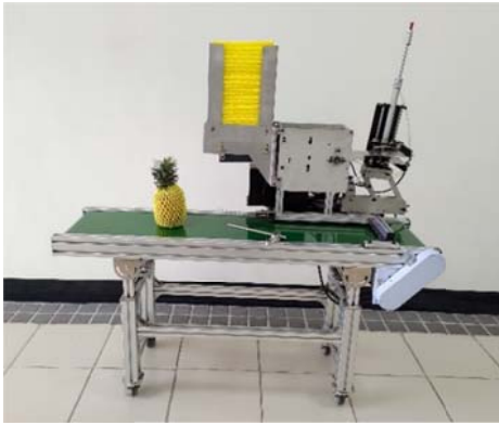
鳳梨果實網袋包裝機械
