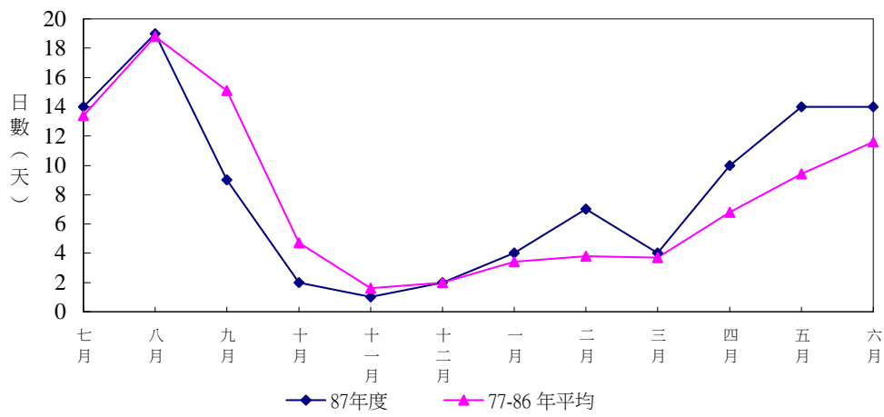
圖4、高雄區農業改良場87年度各月降雨日數
