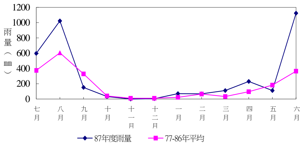
圖 5、高雄區農業改良場各月降雨量
