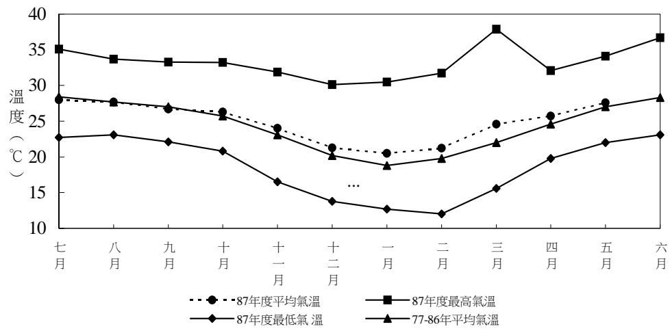
圖1、高雄區農業改良場87年度各月平均氣溫
