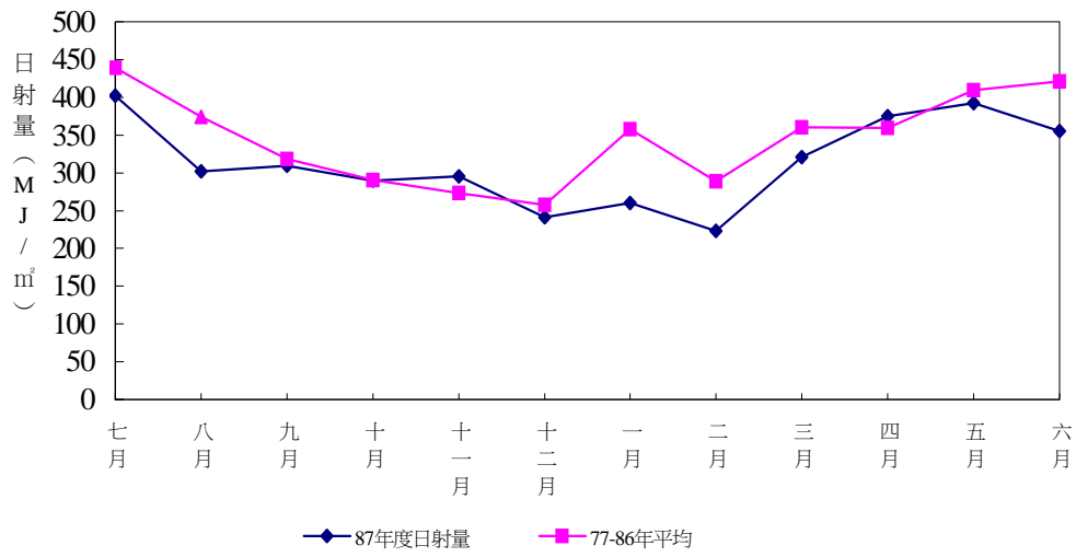
圖3、高雄區農業改良場87年度各月累計日射量
