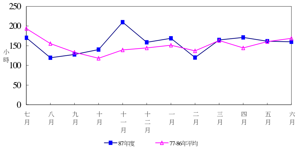
圖2、高雄區農業改良場87年度各月累計日照時數
