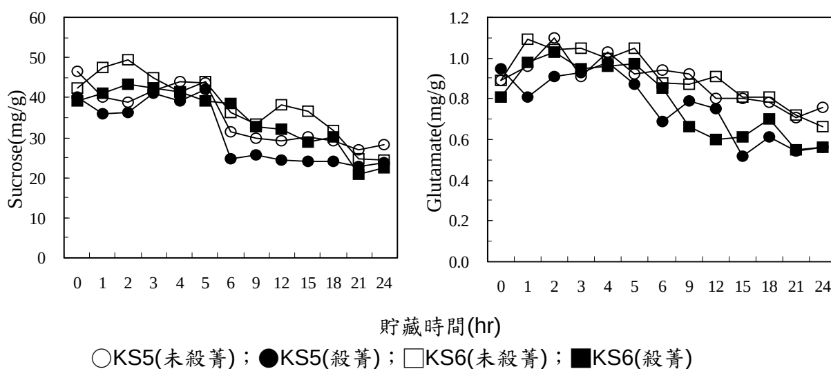
圖 2. 毛豆採收後不同貯藏時間之加工冷凍豆莢之品質分析
