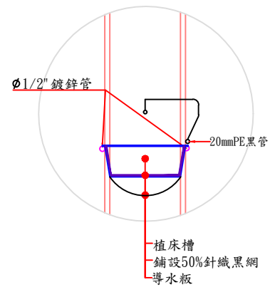
植床詳圖
