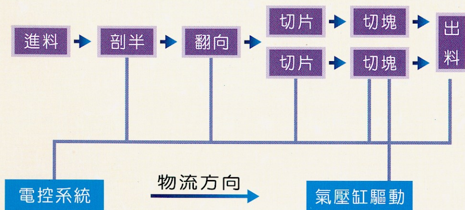
圖五 蔬果切割加工一貫化作業機流程
