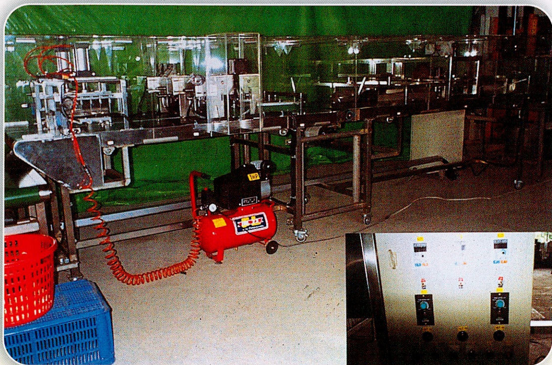
圖四 蔬果加工一貫作業化機械側視圖
