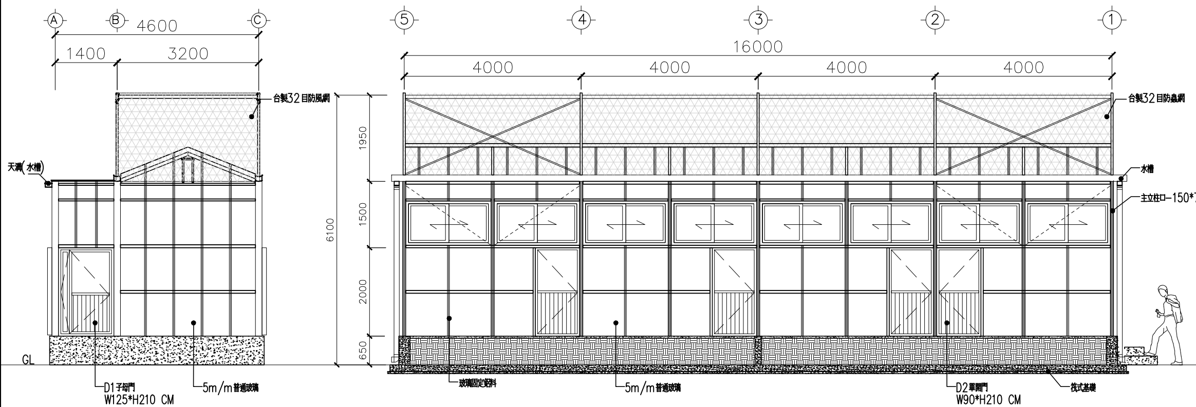
1、5 Line 立面圖 S=1/80
