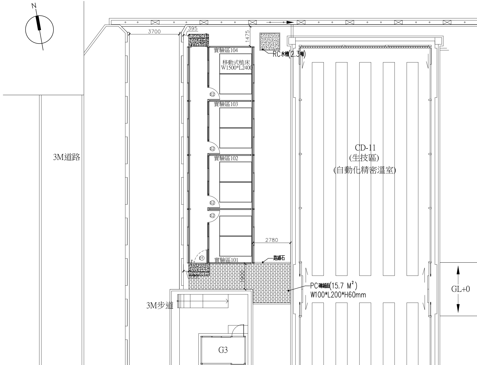
全區配置圖 S=1/120
