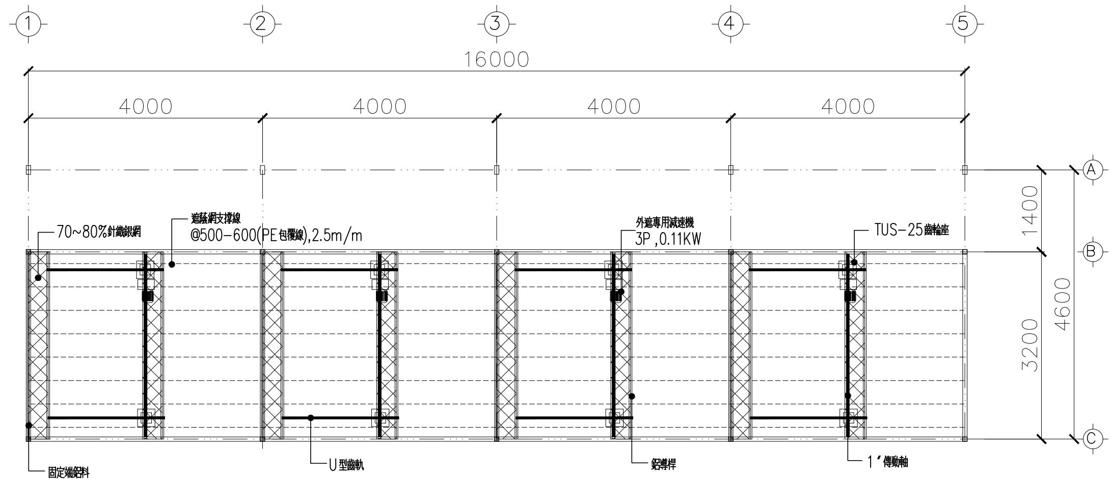
外遮蔭懸掛式驅網系統圖 S=1/60
