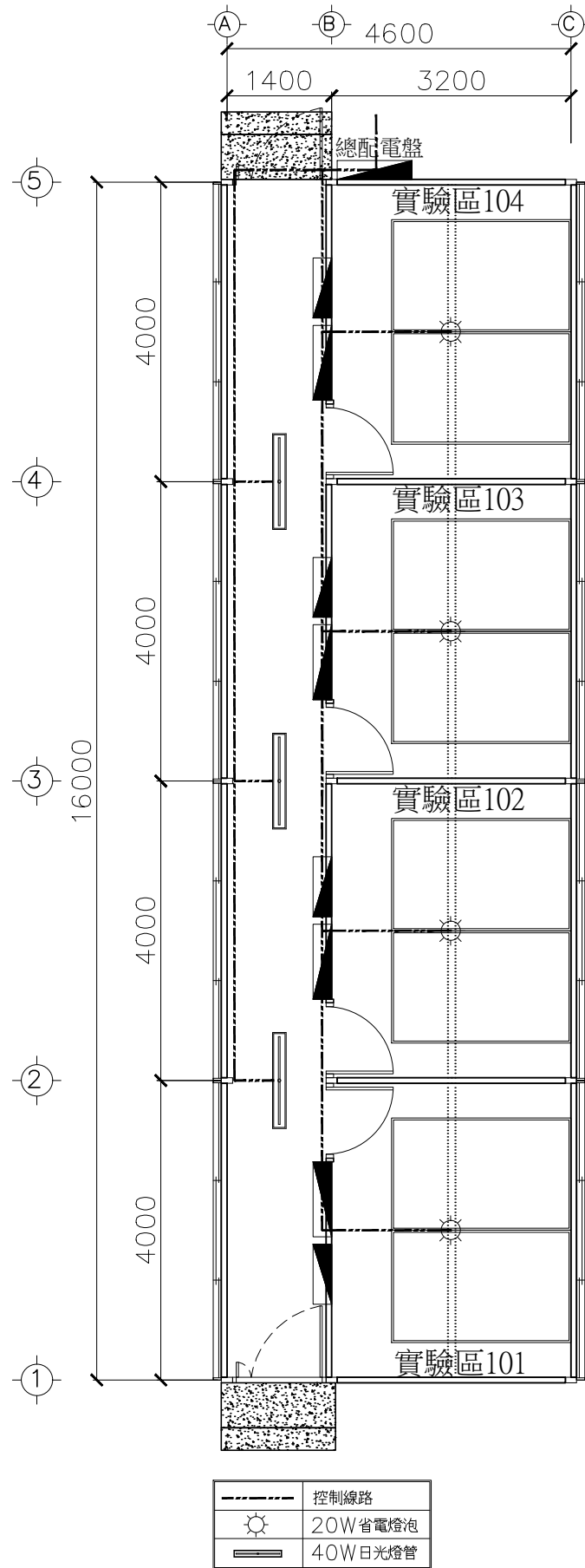
一般照明配置圖 S=1/80
