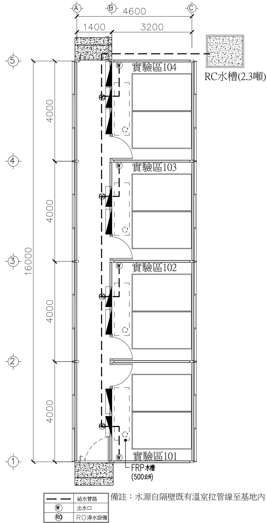
一般用水配置圖 S=1/80
