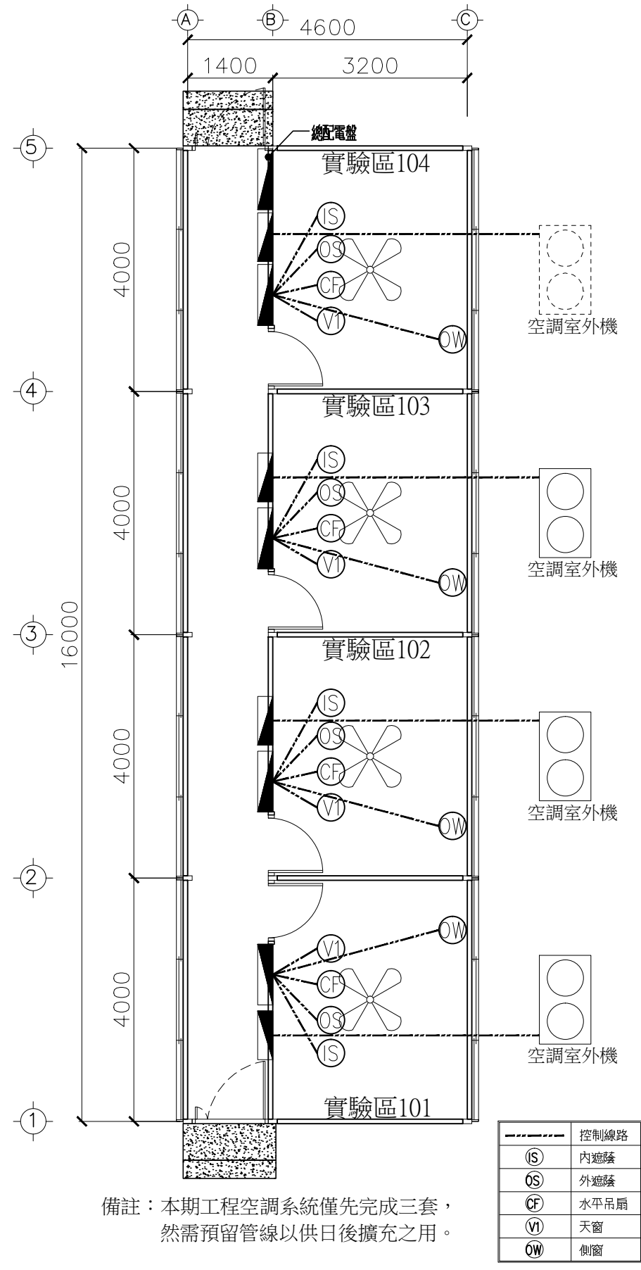
溫室環境設備對應配置圖 S=1/80
