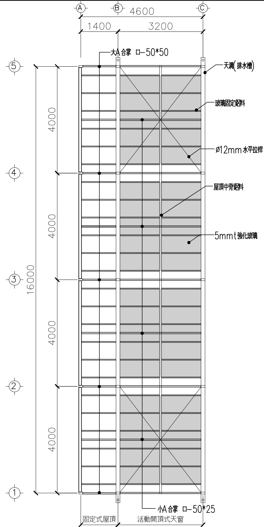
屋頂平面圖 S=1/80
