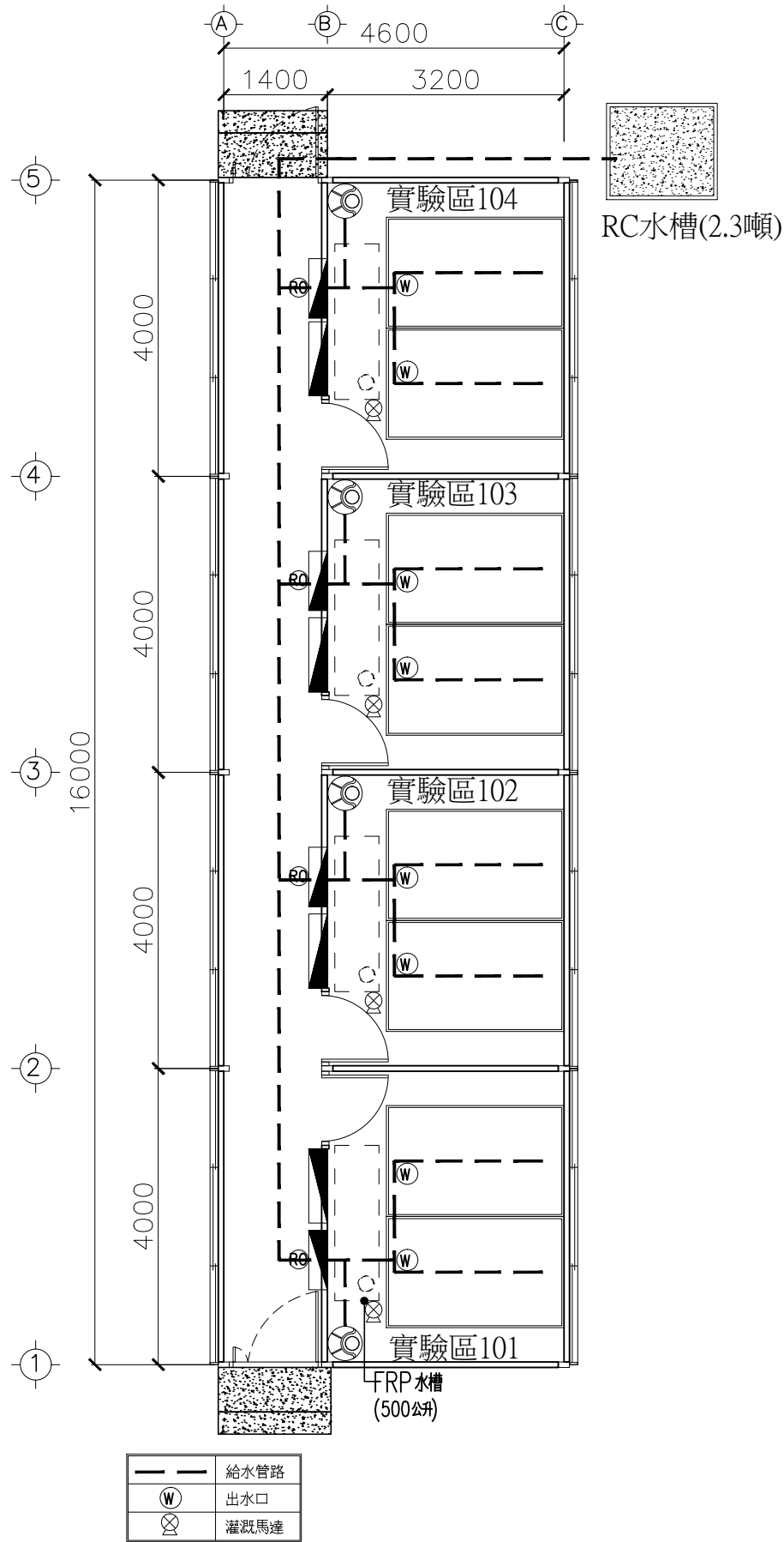
滴灌系統配置圖 S=1/80
