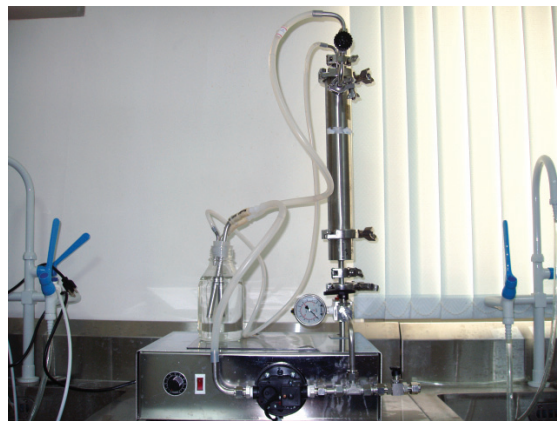
▲水解液NF膜管過濾分離
