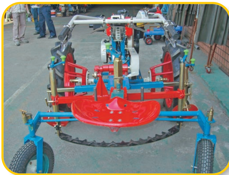
▲ 圖7. 自走式洋葱挖掘機正視
