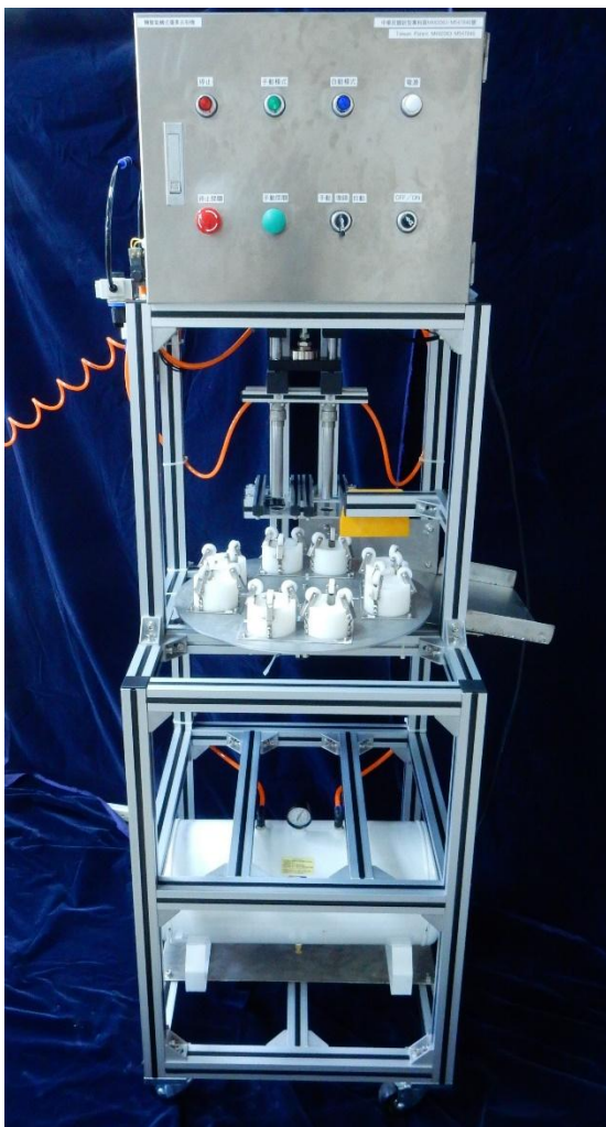
轉盤氣輔式棗果去籽機
